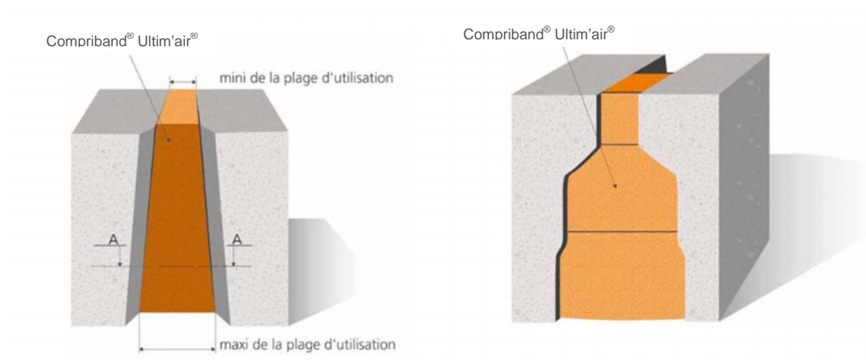
Croquis 6.1 : Étanchéité avec plage d'utilisation
