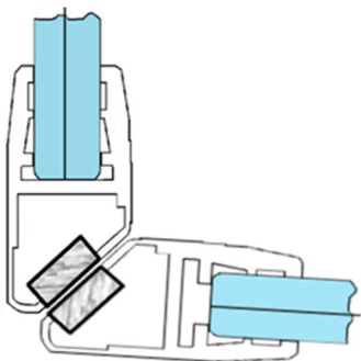
PORTE 90°
