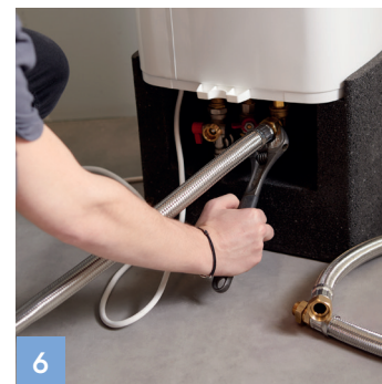
6 Raccorder les flexibles d'EasySwitch aux arrivées d'eau
