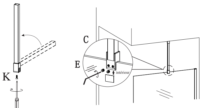
Barre de stabilisation universelle : pose horizontale ou verticale Horizontal or vertical fastening bar
