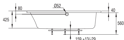
Vidage baignoire fourni
