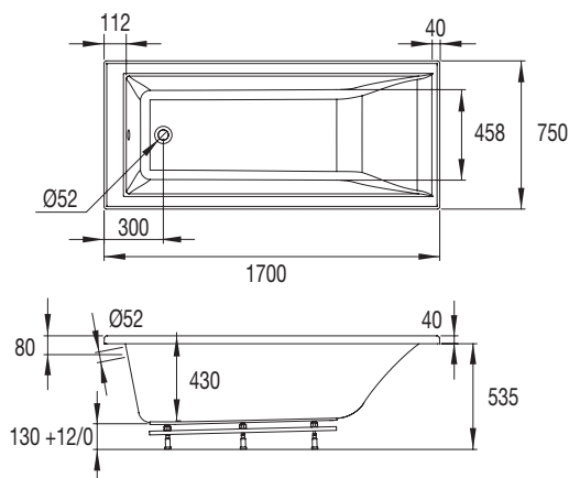
Vidage baignoire fourni
