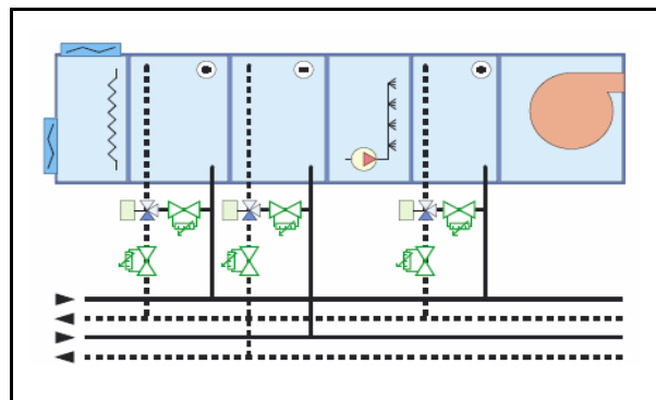
Equilibrage des batteries de traitement d'air
