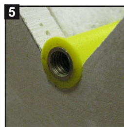
5 Débloquer l'écrou, dévisser le contre-écrou. La cheville est prête à recevoir la pièce à fixer.
