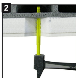
2 Enfoncer la cheville entièrement au ras de la plaque de plâtre à l'aide d'un marteau.
