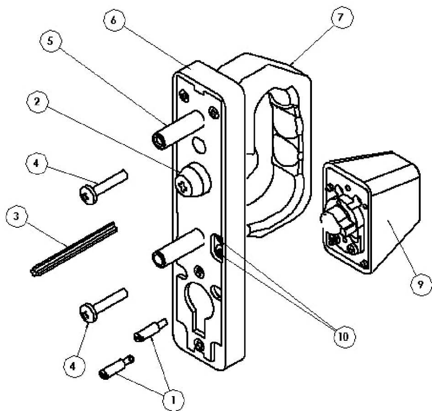
Fig.1 PROTECTEUR ET SUPPORT POUR CYLINDRE FICHET DE TYPE AP89
