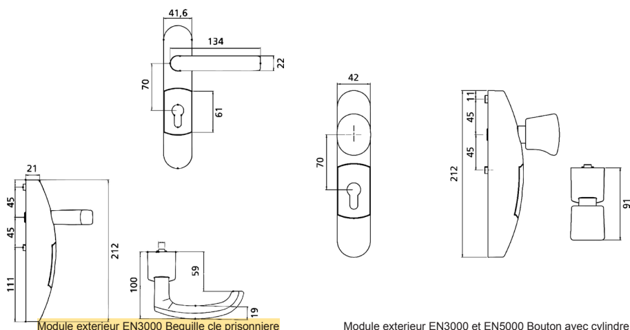
Module extérieur EN3000 Bequille cle prisonniere
