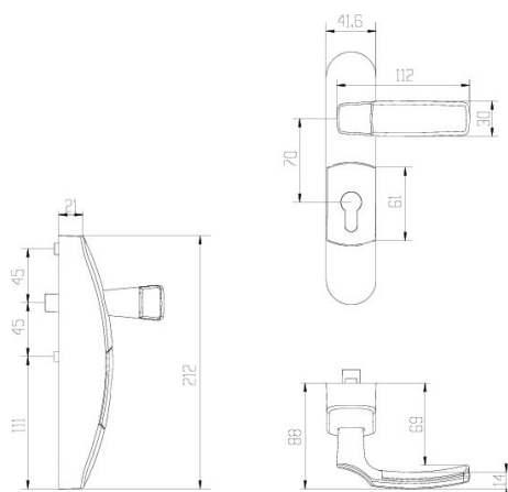
Module extérieur EN5000 Béquille avec cylindre
