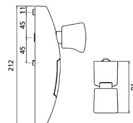
Module extérieur EN3000 et EN5000 Bouton avec cylindre
