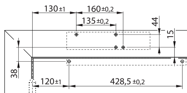
Montage sur dormant côté opposé aux paumelles
