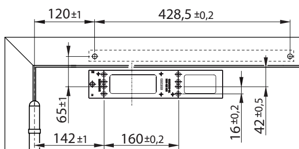
Montage sur ouvrant côté paumelles avec plaque de montage
