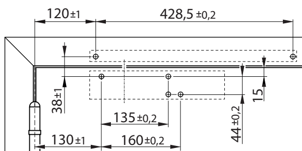
Montage sur ouvrant côté paumelles
