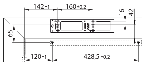
Montage sur dormant côté opposé aux paumelles avec plaque de montage
