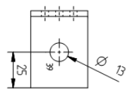
Figure A.83 hold-down 8799 5004 1E
