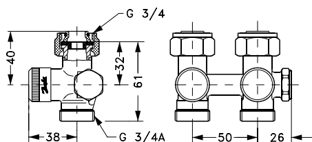
RLV-K droit, pour sortie radiateur G3/4" mâle
