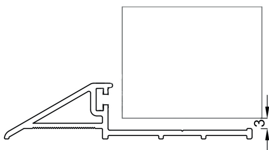
Coupe sur ouvrant
