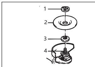
1. Bride extérieure 2. Meule à centre concave 3. Bride intérieure 4. Arbre d'entraînement
