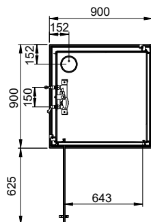
CARRÉ / VIERKANT (KCDJ) 90x90
