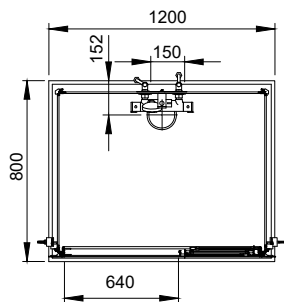
RECTANGULAIRE / RECHTHOEK (KCDTrw) 80x120
