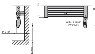
VERSION ELECTRIQUE à liaison infrarouge
