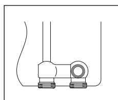
Pour radiateurs à robinetterie intégrée G 3/4 M selon DIN EN 16313 (« eurocône »)
